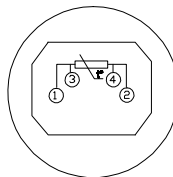
схема расключения колодки TCM 012.50 4х-пров.
