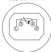
схема расключения колодки TCM 012.50 4х-пров.
