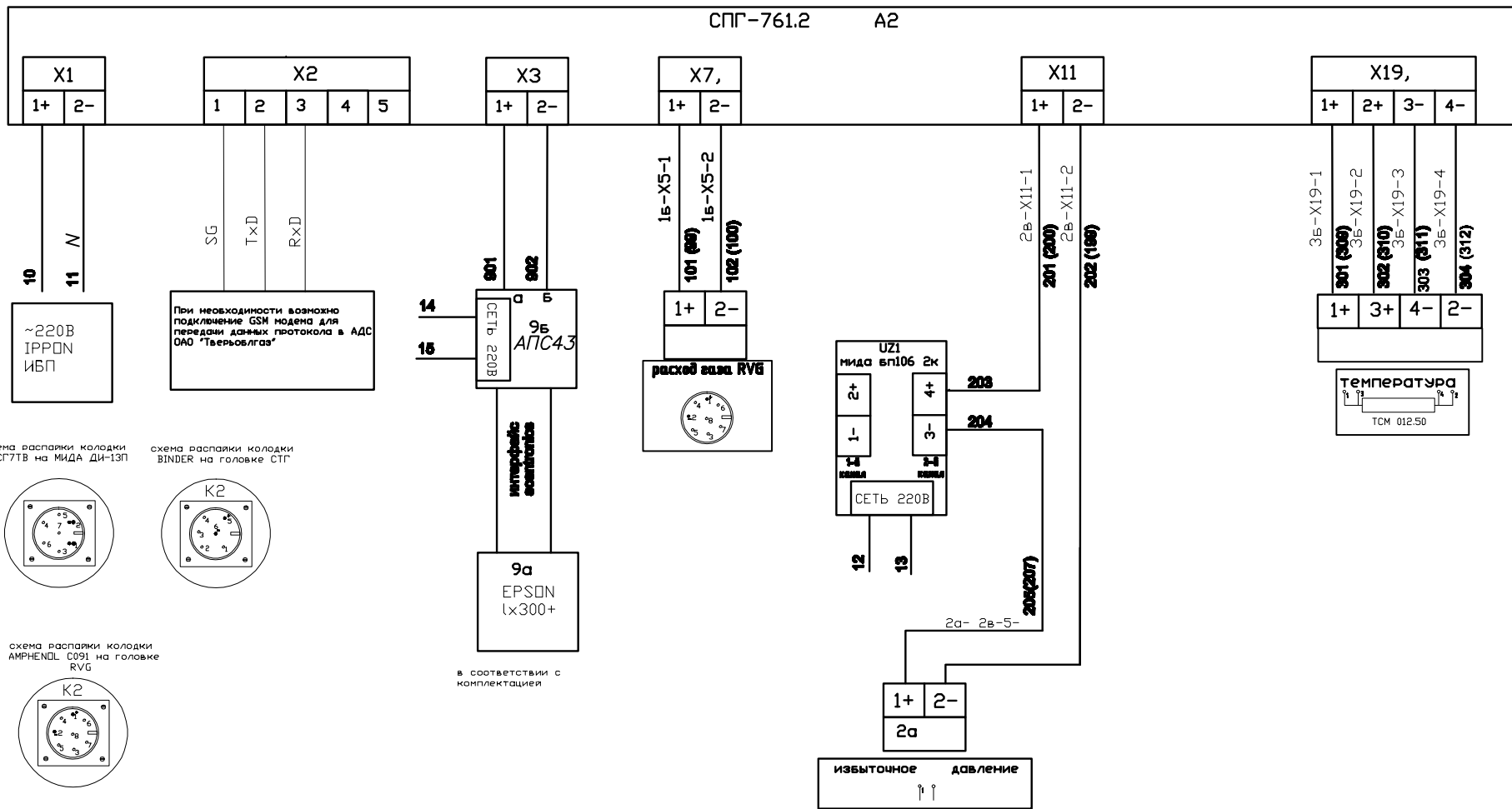
схема расключения колодки TCM 012.50 4х-пров.
