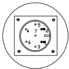
схема расправки колодки РСГ7ТВ на МИДА ДИ-13П
