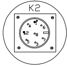
схема расправки колодки AMPHENOL C091 на головке RV6
