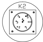
схема расправки колодки BINDER на головке СПГ
